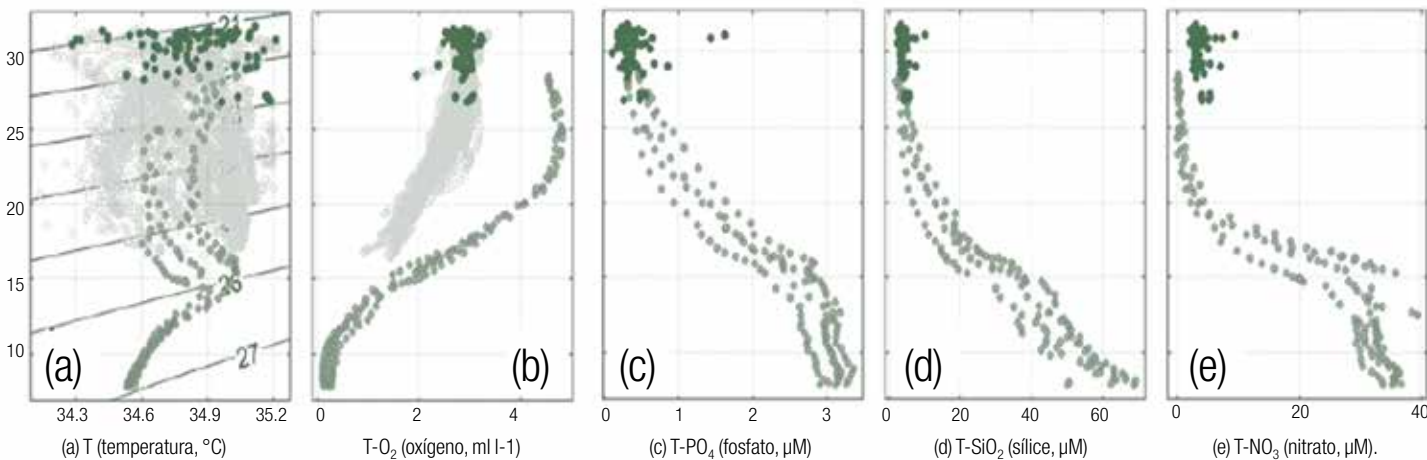
Figura 7. Diagramas de temperatura, salinidad, oxígeno, fosfato, sílice y nitrato.
