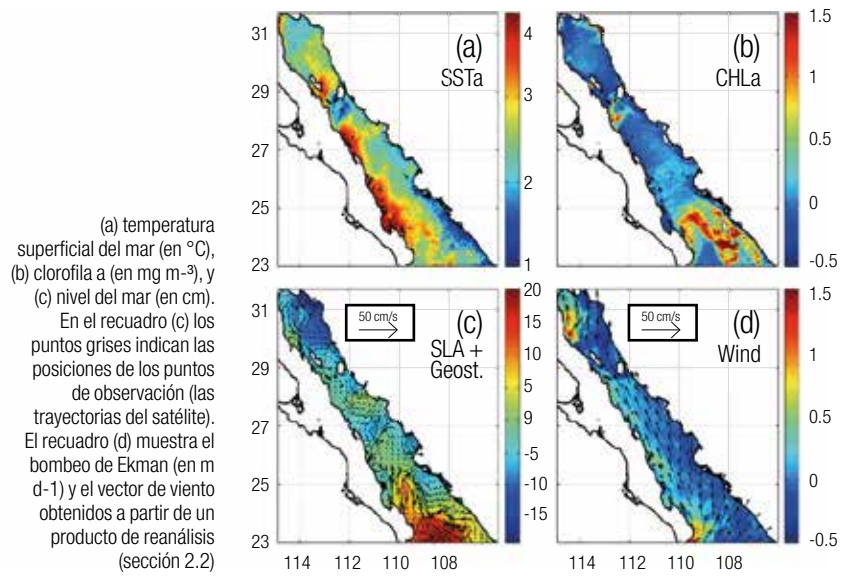
Figura 2. Anomalías con su respectiva velocidad geostrofica, obtenidos a partir de datos satelitales para agosto de 2015 (vea Sección 2.2).
