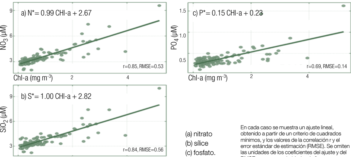
Figura 6. Relación lineal entre clorofila-a, nitrato, sílice, y fosfato.
