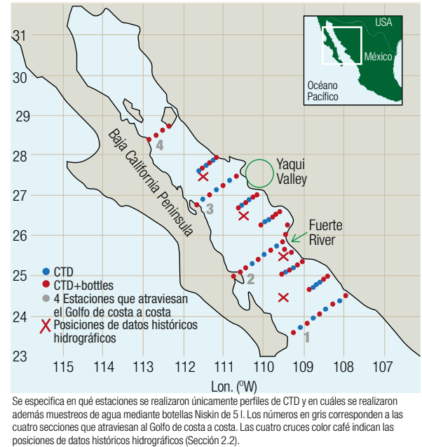
Figura 1. Posición de 65 estaciones hidrográficas realizadas en el muestreo Greenpeace-FAN
